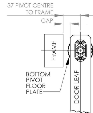
DOOR OPEN 90°
